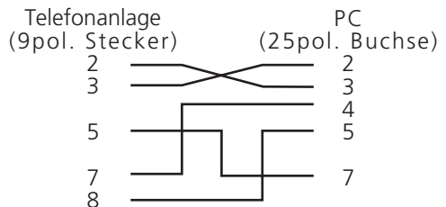
Anschlussbelegung des PC-Kabels
